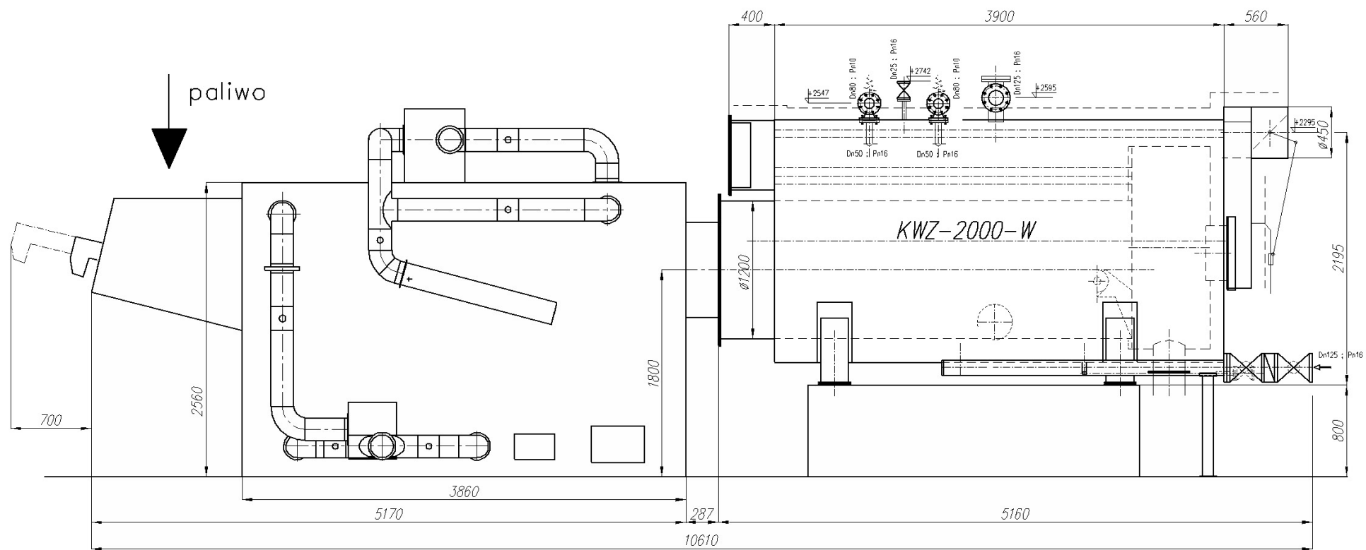
Kocioł wodny z przedpaleniskie-ruszt schodkowy Moc kotła – 2MW Paliwo – biomaso-zrębki
