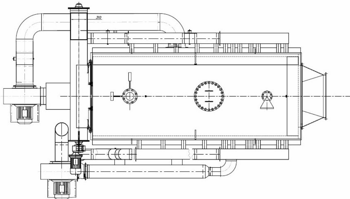
Kocioł wodny z rusztem schodkowym Moc kotła - 2MW Paliwo - biomasa - zrębki
